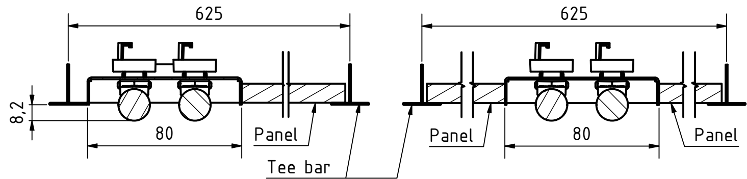
A-A ( 1 : 2 )
